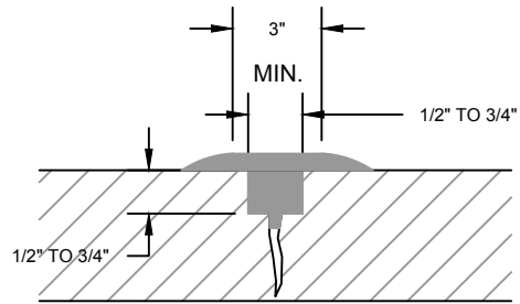
(D) STANDARD RECESSED OVERBAND
